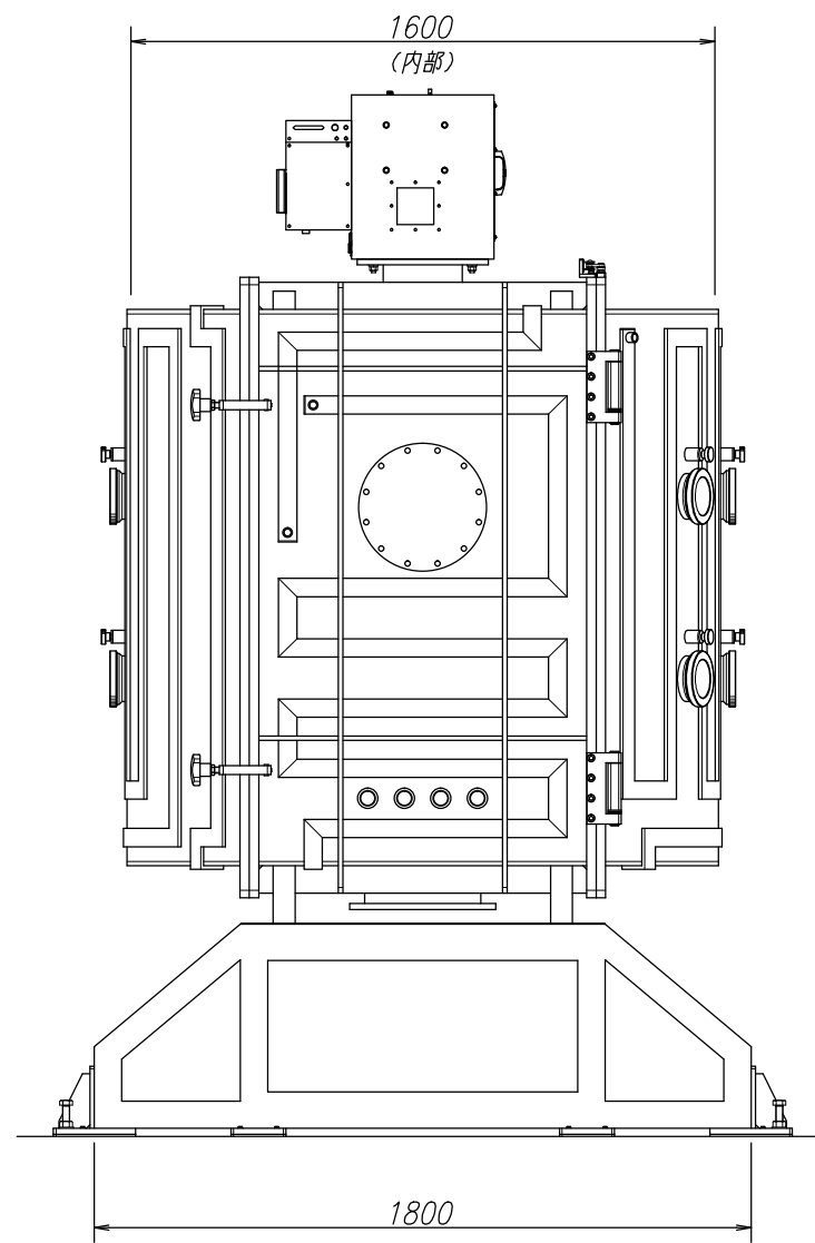
真空装置（左側面）
