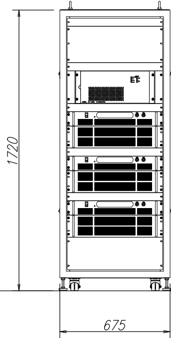
電源収納盤
