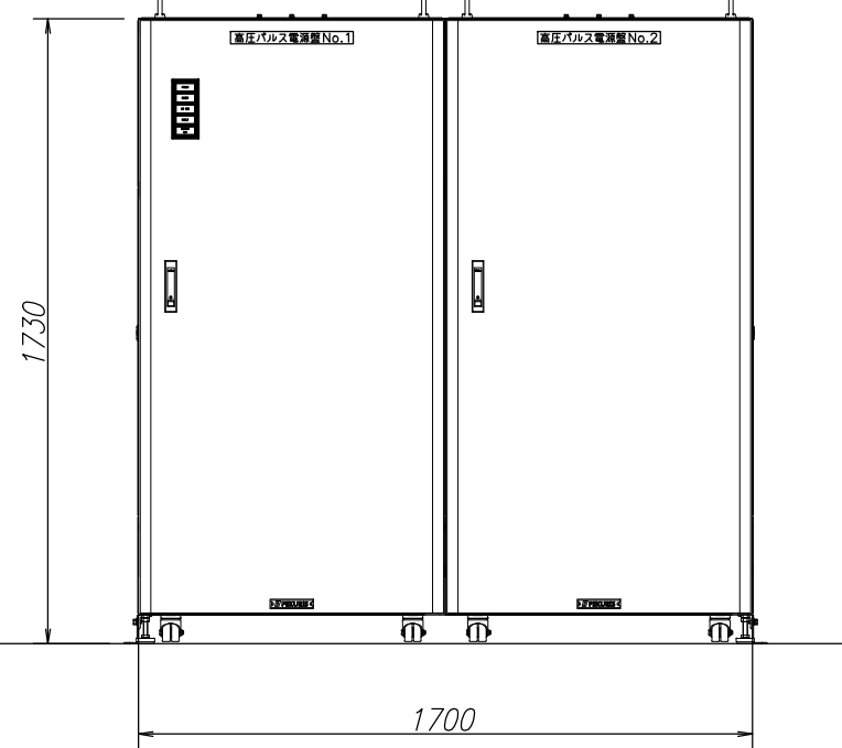
高圧パルス電源盤
