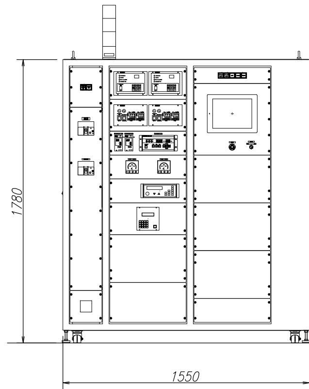
操作盤
