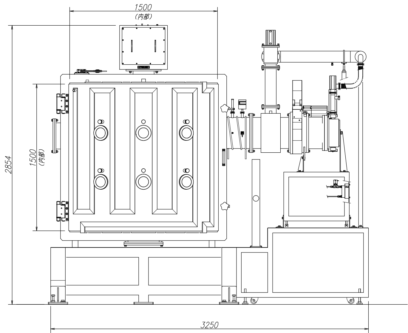
真空装置（正面）
