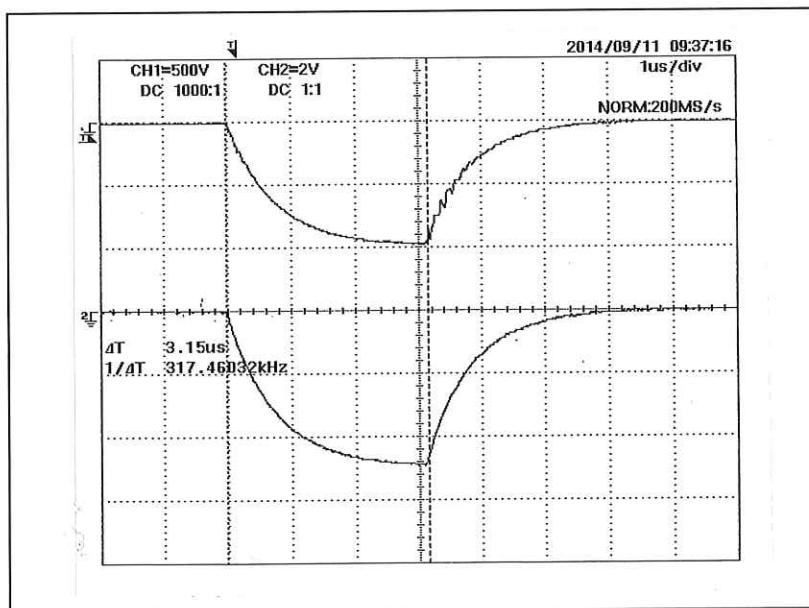
波形4 抵抗負荷試験条件2 R_L \doteq 20\Omega 出力電圧 CH1 500V/div 出力電流 CH2 20A/div
