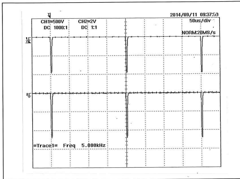
波形3 抵抗負荷試験条件2 R_L \doteq 20\Omega 出力電圧 CH1 500V/div 出力電流 CH2 20A/div
